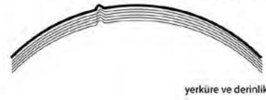
yerküre ve derinlik
