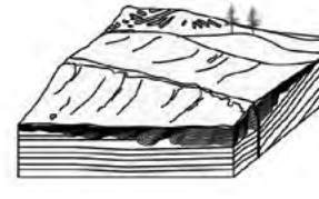
Tabaka tipi traverten morfolojisinin blok diyagramındaki şematik görünümü
