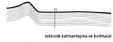
tektonik katmanlaşma ve kırılmalar
